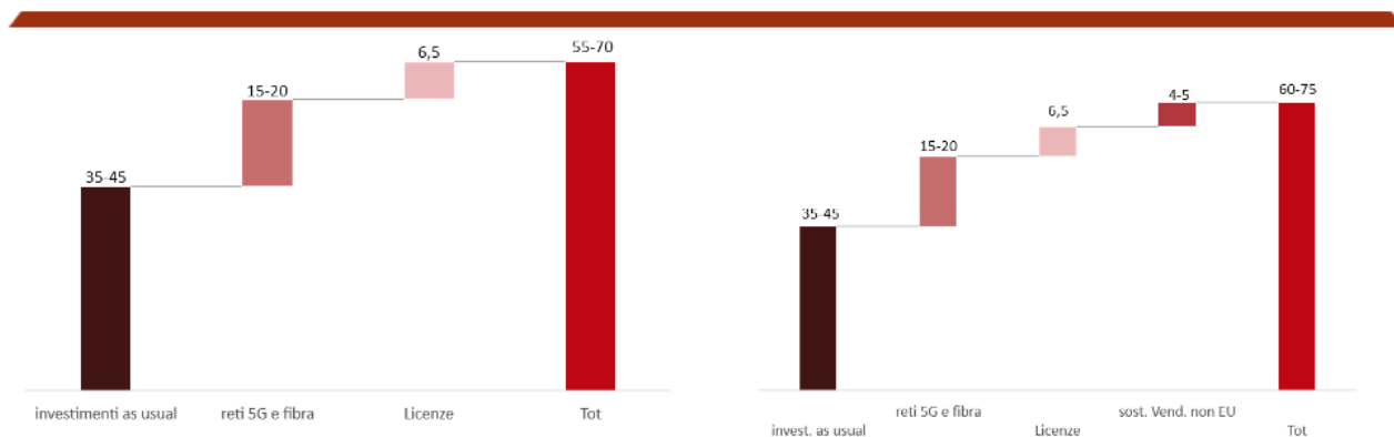
FIGURA 4.2 Stima investimenti necessari per l'implementazione delle reti 5G in Italia (in € mld, 2019-2025)
