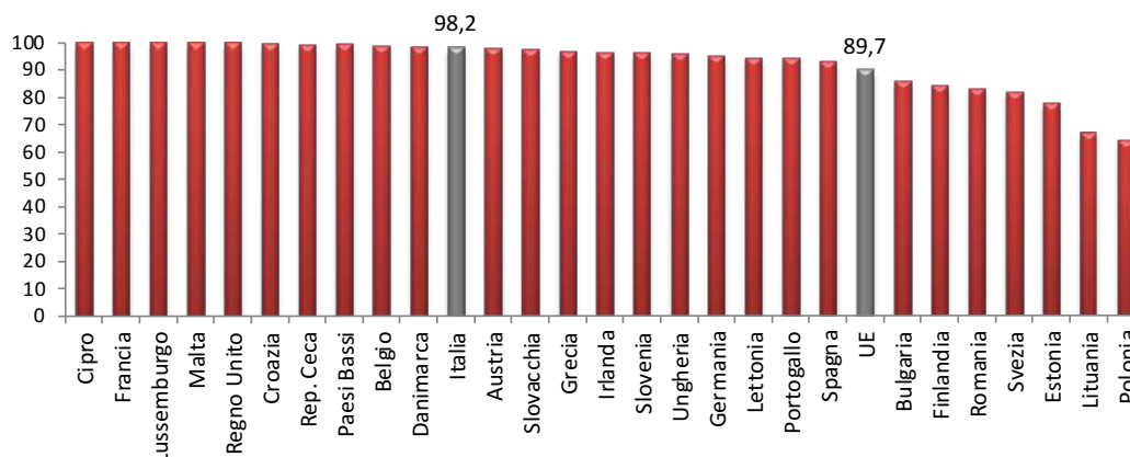
Figura 2.7 Copertura VHCN nelle aree rurali (valori in %, 2020)
