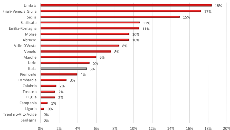
Figura 6.11 Comuni con siti FWA collaudati positivamente (% su totale comuni previsti; 31 agosto 2021)
