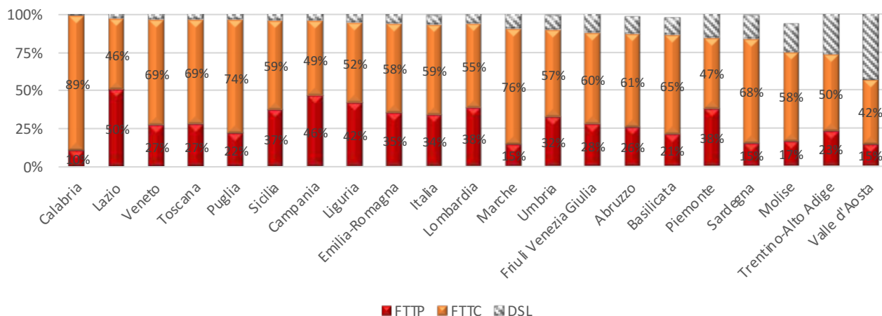
Figura 6.2 Copertura provinciale (% famiglie coperte, dicembre 2020)
