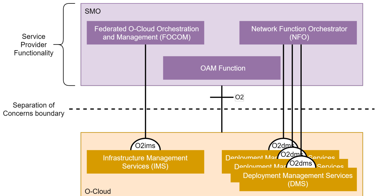
Abbildung 13: Aufteilung der O2-Schnittstelle in Service Bases Interfaces (Ref. [25])
