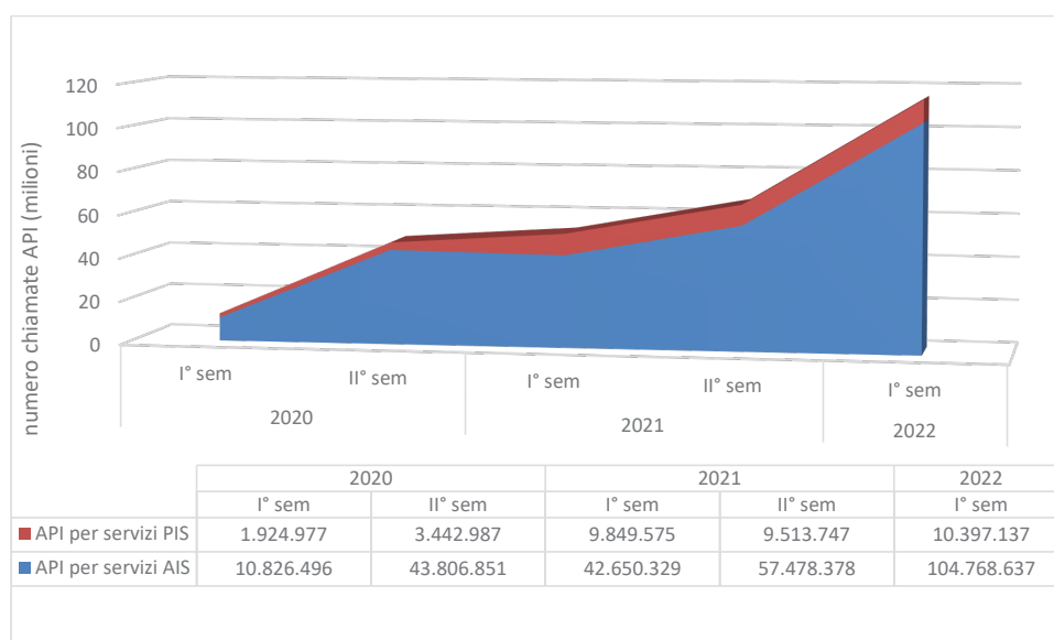
Figura 12 – Numero delle chiamate API per tipo di servizio (PIS/AIS)
